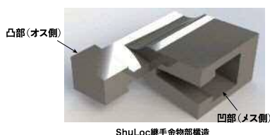
ShuLoc継手金物部構造
